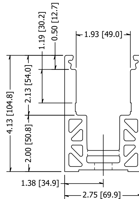
VIEW A-A
